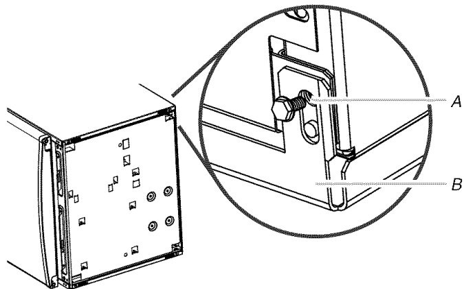
A. Trou arrière du réfrigérateur/congélateur convertible B. Bride de roulette
