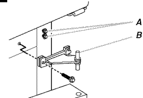
A. Vis de charnière à tête hexagonale de \frac{5}{16} " B. Charnière centrale
