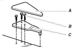
A. Couvercle de la charnière supérieure B. Vis de charnière à tête hexagonale de \frac{5}{16} " C. Charnière supérieure
