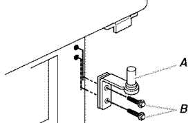
A. Bisagra inferior B. Tornillos de cabeza hexagonal para bisagra de 5/16"
