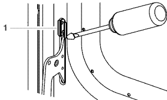
1. Door Stop Clip
