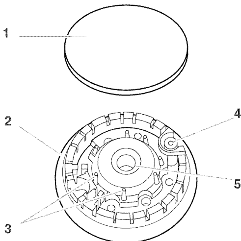
1. Tapa del quemador 2. Base del quemador 3. Espigas de alineamiento 4. Encendedor 5. Abertura del tubo de gas
