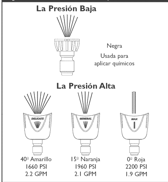
Figura 35 — Rocíe los Modelos del Boquilla
