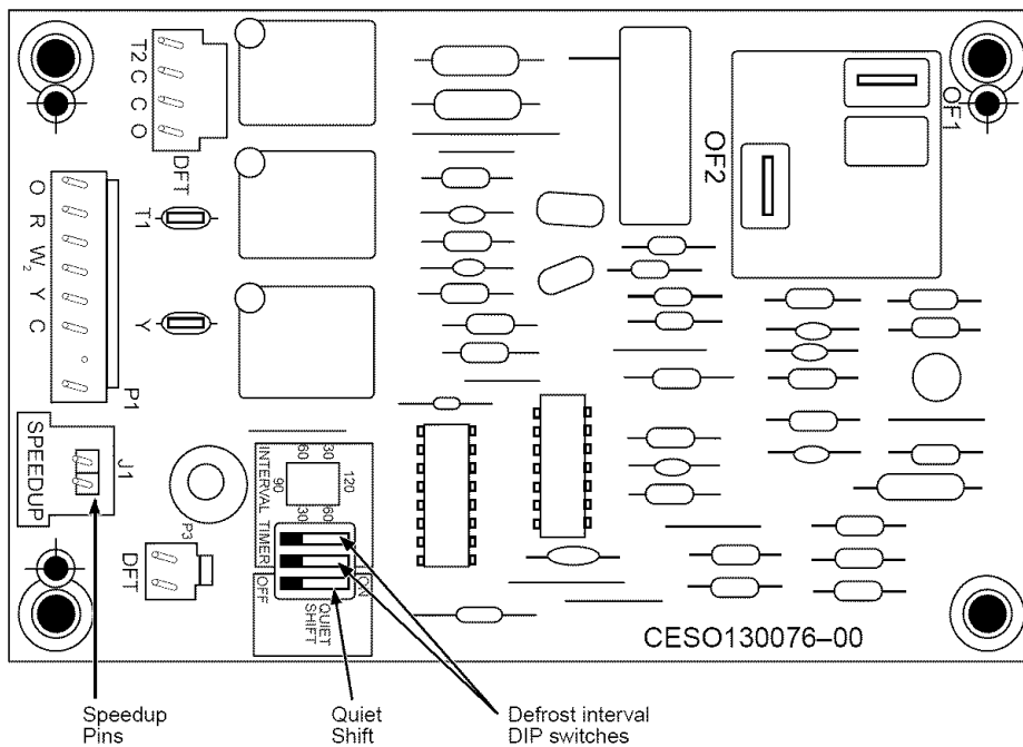
Fig. 14—Defrost Control
