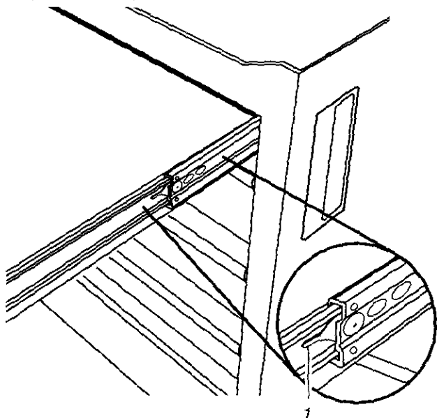
1. Palanca
