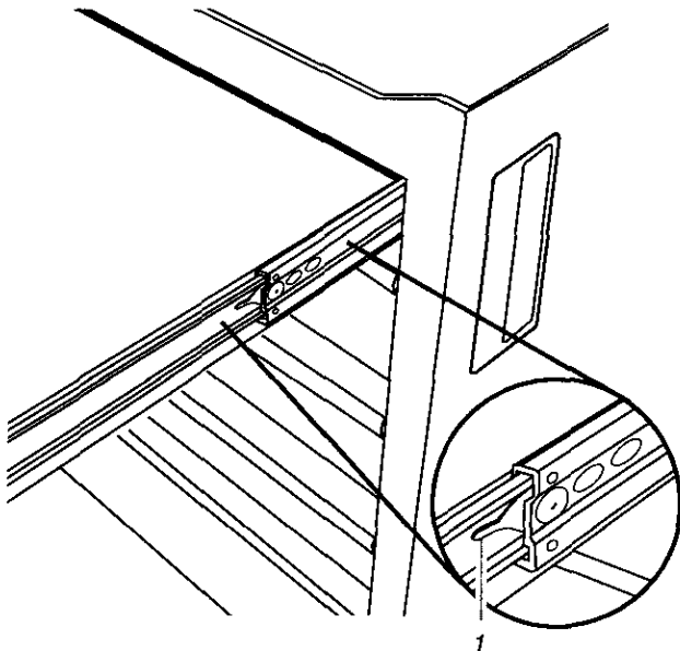
1. Manette
