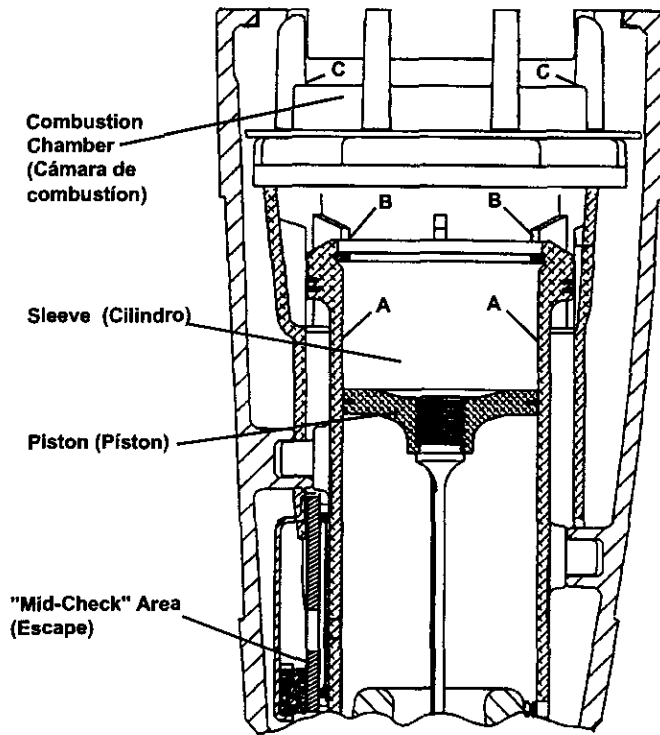
Motor Assembly Conjunto del Motor
