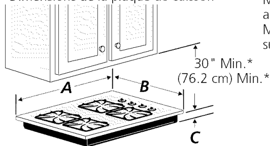
Dimensions de la plaque de cuisson
