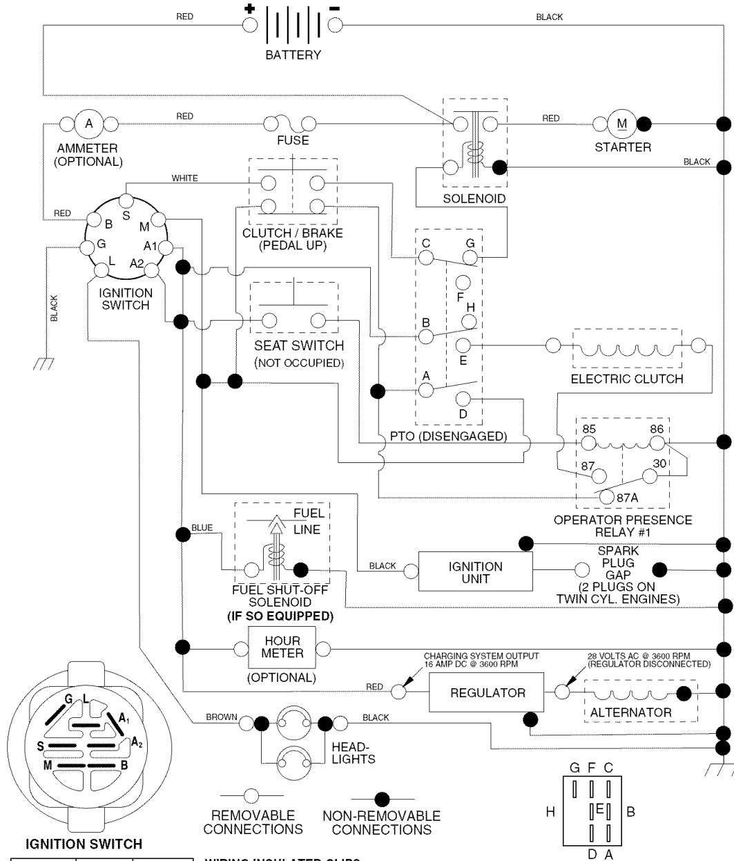
PTO SWITCH
