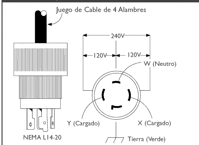
Figura 14 — 120/240 Volt AC, 20 Amp, Receptáculo de Seguridad
