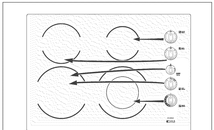
Parrilla de cocinar 30" - Ubicación de los Elementos Superiores Radiantes y de los Controles Figure 1
