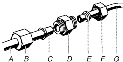
A. Tubería de agua del refrigerador B. Tuerca C. Bulbo D. Acoplamiento E. Férula F. Tuerca G. Línea de agua de la casa
