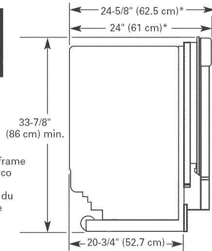
Side view Vista lateral Vue latérale
