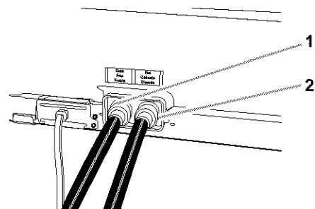
1. Électrovanne d'alimentation - bleu = eau froide 2. Électrovanne d'alimentation - rouge = eau chaude
