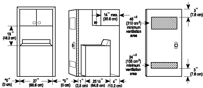
1. Vista frontal 2. Vista lateral 3. Puerta del armario con celosías de ventilación
