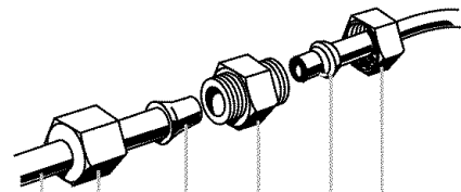
A. Tubería de agua B. Tuerca (provista) C. Bulbo D. Acoplamiento (adquirido) E. Férula (adquirida) F. Tuerca (adquirida)
