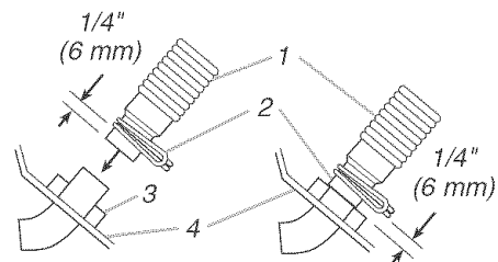
1. Tuyau d'évacuation 3. Butée nervurée 2. Bride 4. Caisse
