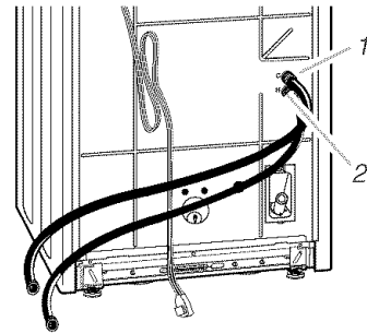
1. Electrovanne d'alimentation - bleue = eau froide 2. Electrovanne d'alimentation - rouge = eau chaude
