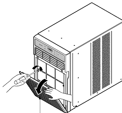
Inlet Grille
