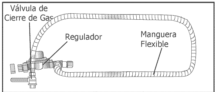
Figura 11: Método con Manguera Flexible
