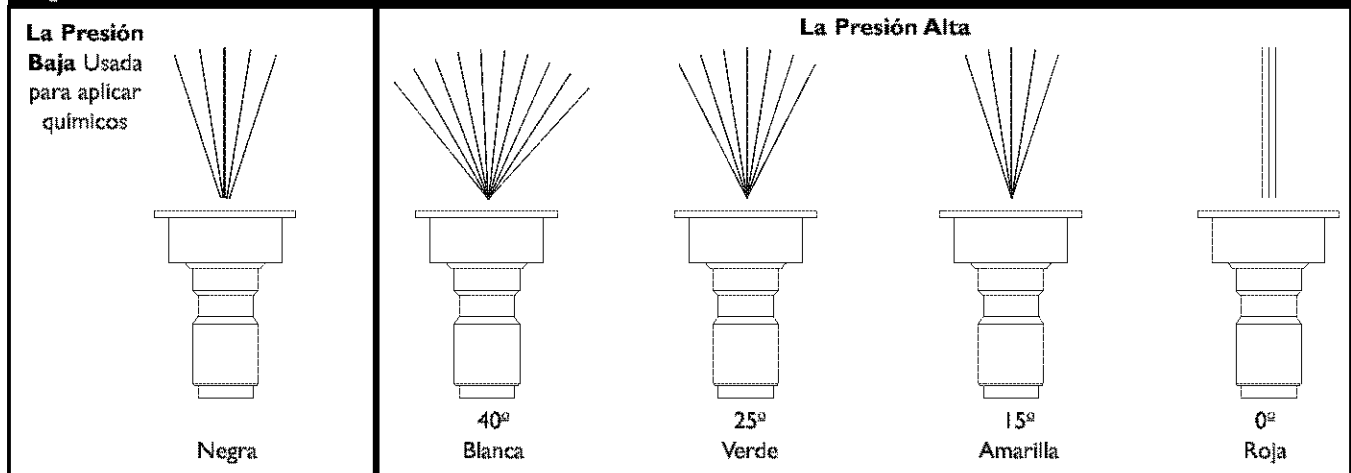
Figura 22 - Punta de Rociado
