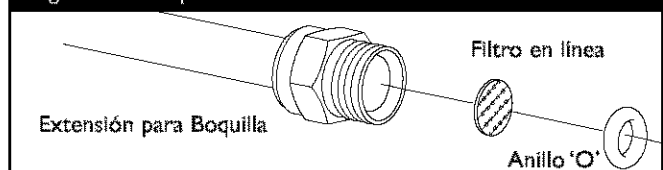
Figura 23 - Limpieza del Filtro
