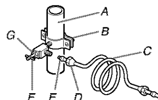
A. Canalisation d'eau froide . E. Bague de compression B. Bride de tuyau F. Robinet d'arrêt C. Tube en cuivre D. Écrou de compression G. Écrou de serrage
