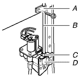
A. Bride du tube C. Écrou de compression B. Tube en cuivre D. Valve d'entrée d'eau
