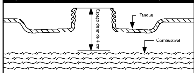
Figura 15 — Espaço de Expansão de Combustível Típico
