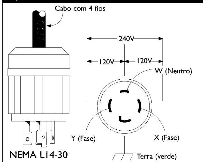
Figura 19 — Tomada com Trava 120/240 V CA, 30 A
