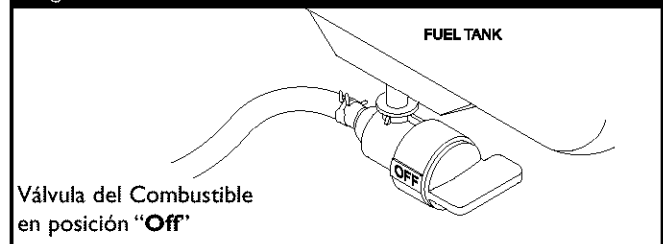
Figura 9 — Válvula de Combustible
