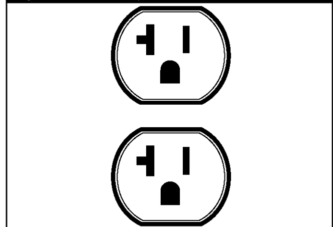
Figura 20 — Tomada Duplex 120 V CA, 20 A
