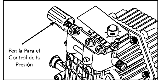
Figura 43 - Perilla Para el Control de la Presión
