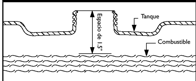
Figura 11 — Espacio Típico para la Expansión del Combustible
