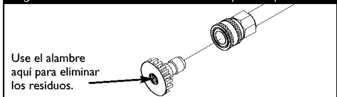
Figura 20 - Mantenimiento de la Extensión para Boquilla
