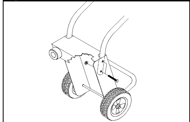
Figura 12 - Conecte la Manecilla al Lavador a Presi n
