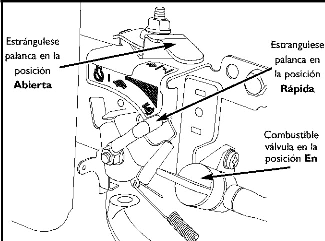
Figura 37 - Controles de Aceleración y de Ahogamiento
