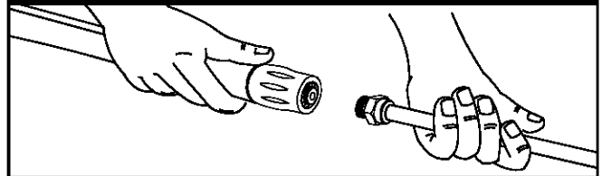
Figura 35 - Conecte la Extensión de la Lanza a la Pistola Rociadora
