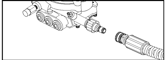
Figura 32 - Conectar la Manguera de Alta Presión a la Toma de Agua
