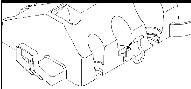
Figura 27 - Colocar el Gancho "J" Hook sobre el Charola Accesoria
