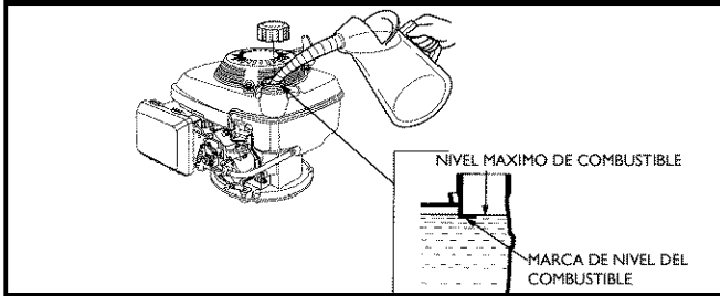
Figura 30 - Añada Gasolina al Tanque de Combustible
