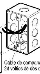
Figura 2 INSTALACIÓN PRECABLEADA
