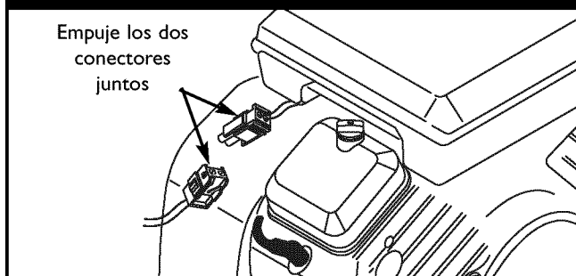
Figura 25 — Conexión del Solenoide de Transferencia de Combustible
