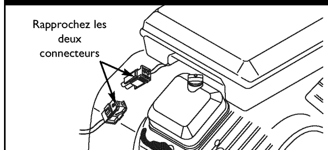
Figure 38 — Raccord de la Solénoïde de Transfert du Combustible
