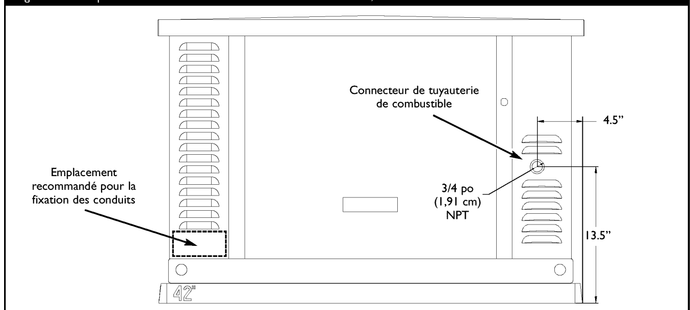
Figure 28 — Emplacement du Combustible et des Éléments de Conduit, Côté Entretien d'Huile de l'Unité
