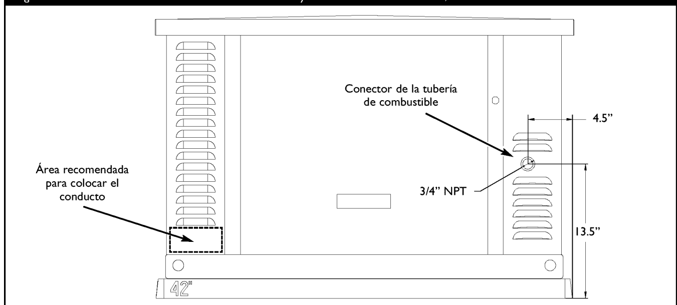
Figura 15 — Ubicaciones de los Accesorios del Conducto y Combustible del Generador, del Lado del Servicio de Aceite de la Unidad
