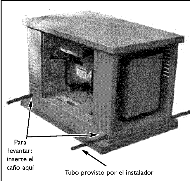
Figura 16 — Ubicación de los Orificios de Elevación
