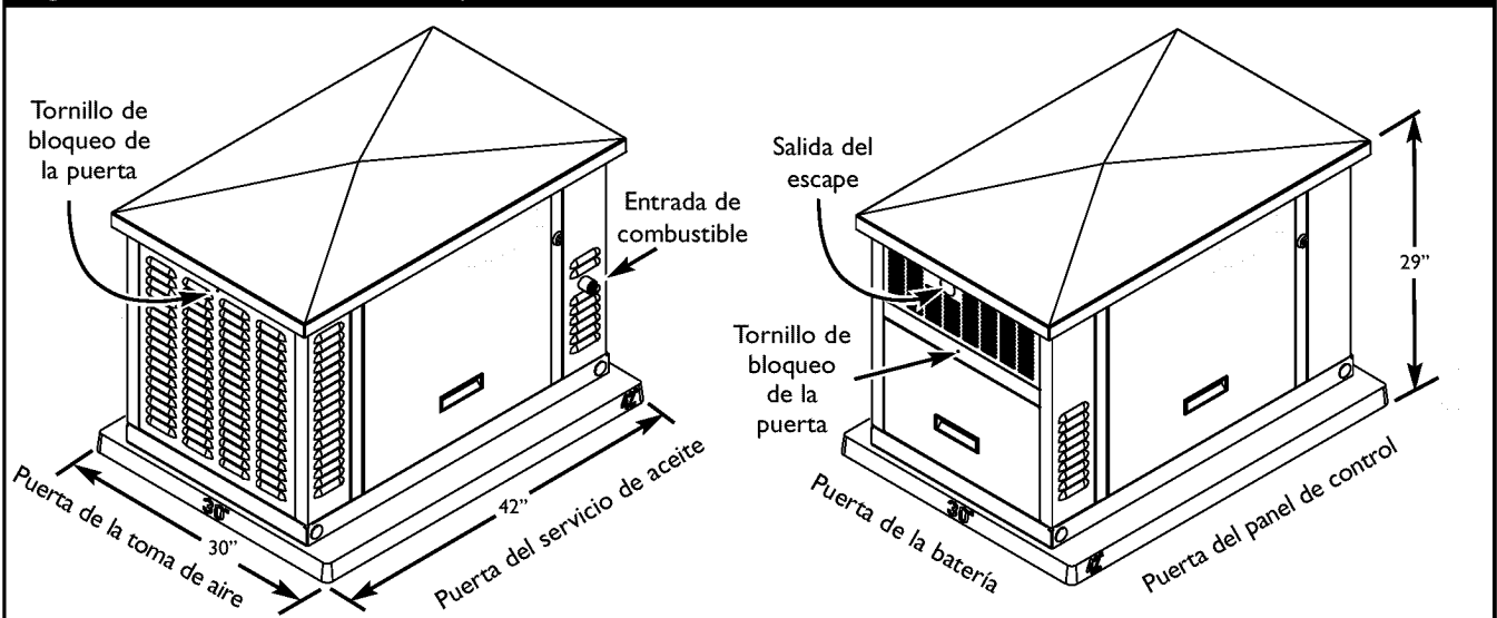
Figura 17 — Puertas de Acceso al Compartimento
