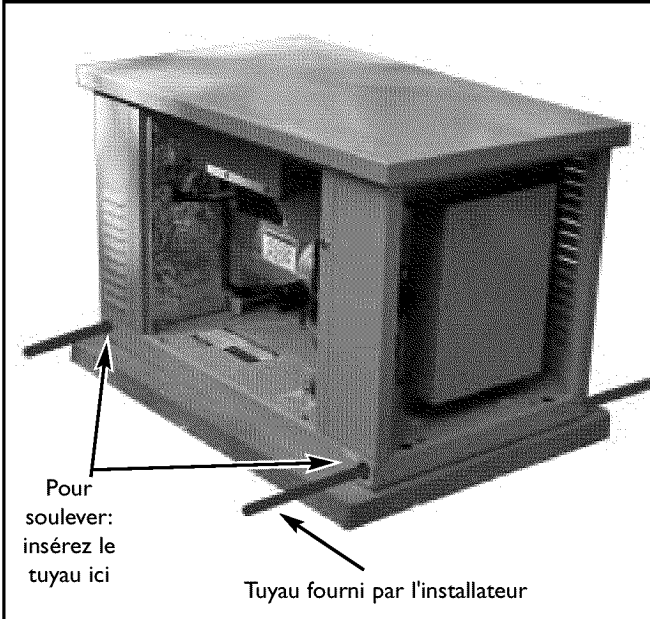
Figure 29 — Emplacement des Trous de Levage
