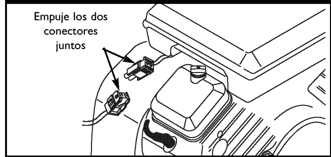
Figura 25 — Conexión del Solenoide de Transferencia de Combustible
