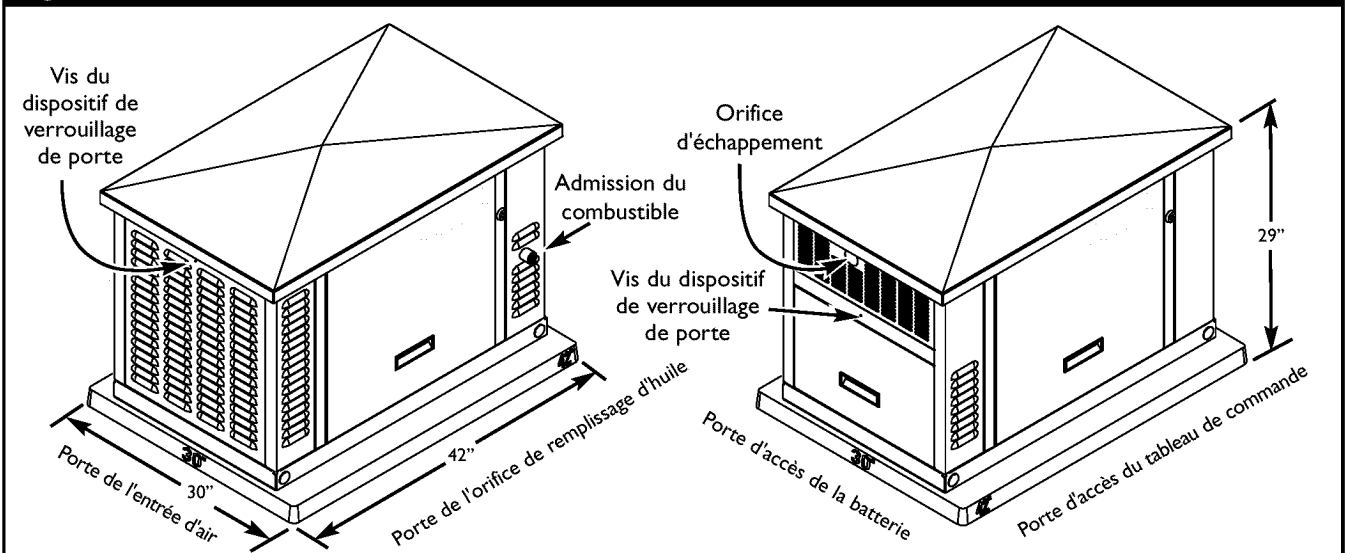
Figure 30 — Portes d'Accès de l'Enceinte
