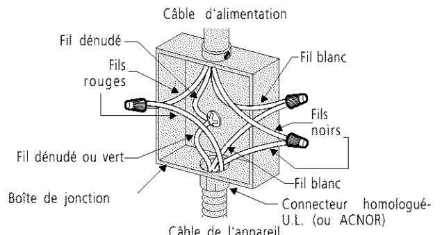
Figure 7 – BOÎTE DE JONCTION À 4 FILS MISE A LA TERRE Modèle 36" avec zone réchaud seulement
