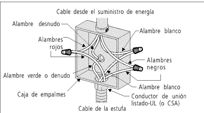
Figura 7 – CAJA DE EMPALME DE 4 ALAMBRES PUESTA A TIERRA Solamente para modelo 36" y zona hornilla
