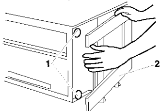
1. Pieds de nivellement 2. Base d'expédition
