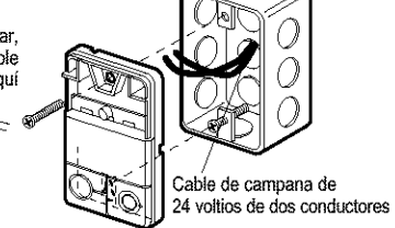
Figura 2 INSTALACIÓN PRE-CABLEADA
