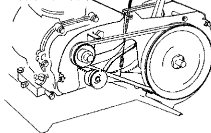
Cable de control de los brazos Abrazadera del cable
