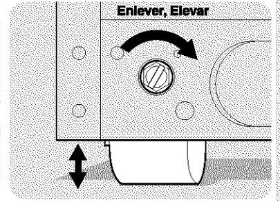
Réglage des roulettes avant. Ajuste de los Rodillos Delanteros.
