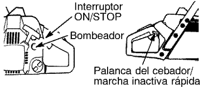
PALANCA DEL CEBADOR/ MARCHA INACTIVA RÁPIDA (VISTA LATERAL)
