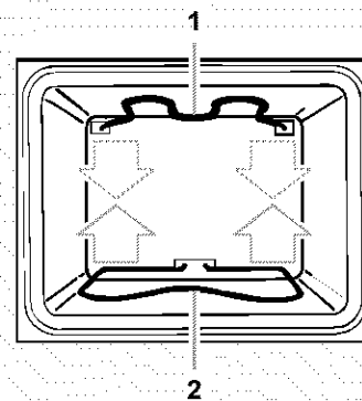
1. Elemento para asar 2. Elemento para hornear
