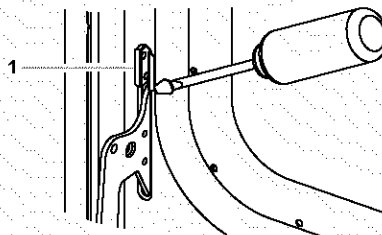
1. Gancho de tope de la puerta
