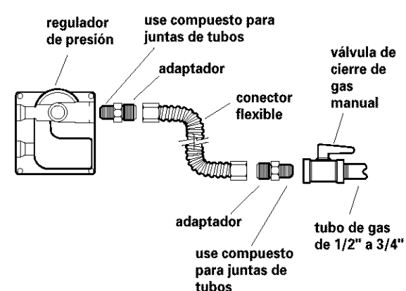
Conexión flexible típica
