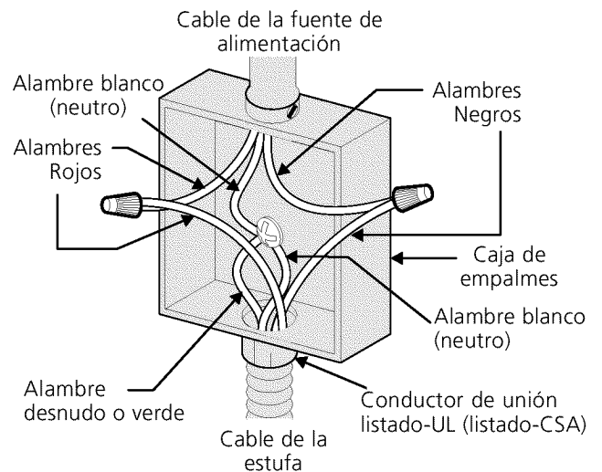
Figura 6 Sistema eléctrico (ejemplo: caja de empalmes) de 3 alambres (a tierra neutra)
