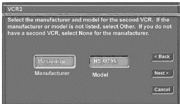
Figure 4. VCR2 menu.
