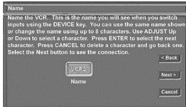
Figure 1. Name menu.
