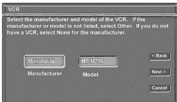
Figure 3. VCR menu.
