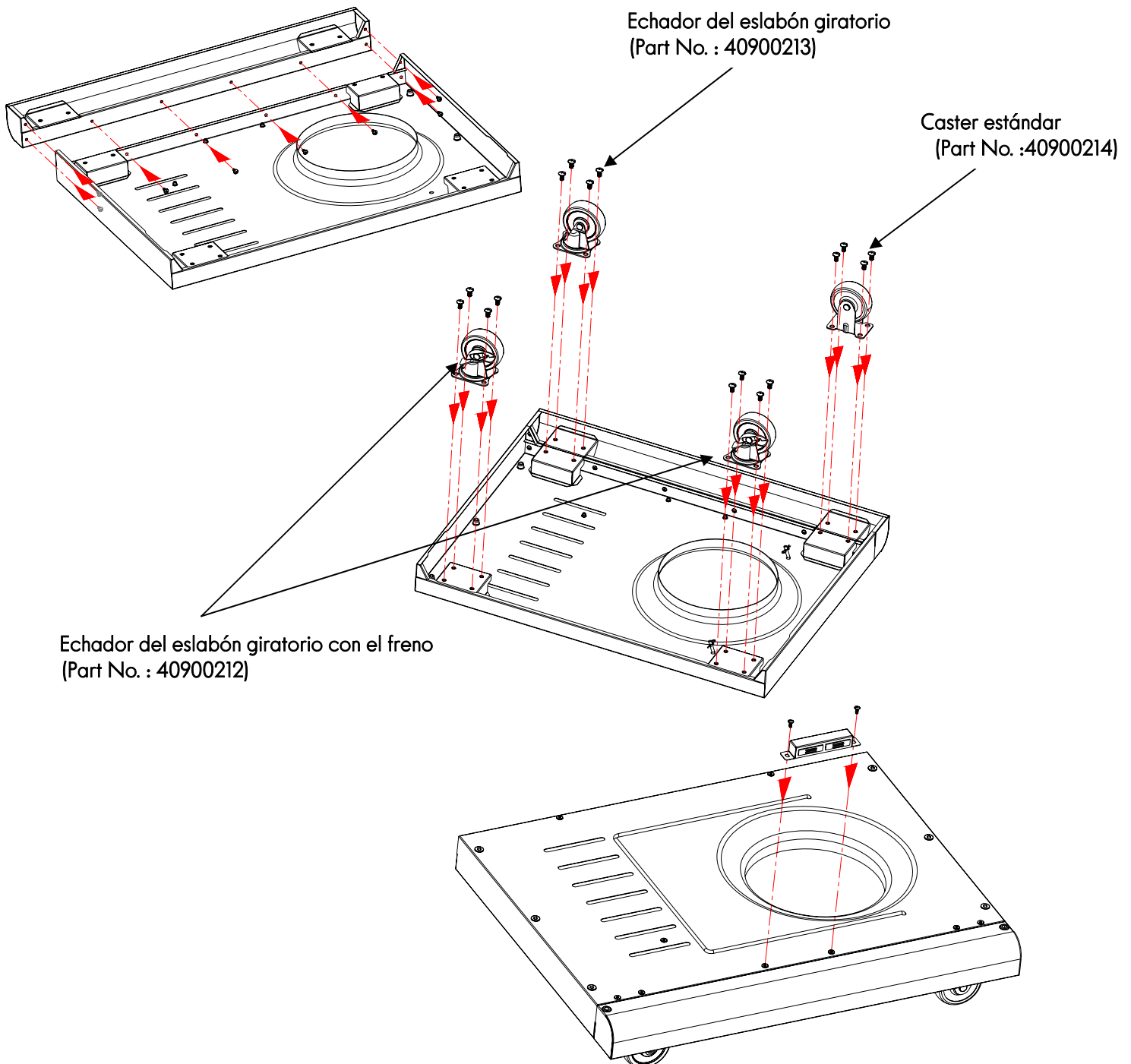
Tornillos M6X13 Qty: 16 pc
