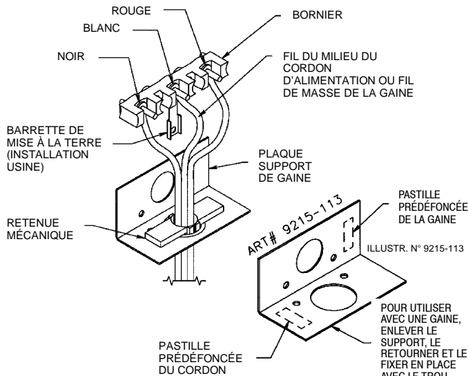
FIGURE 8 INSTALLATION ACCEPTABLE - FICHE À TROIS FILS
