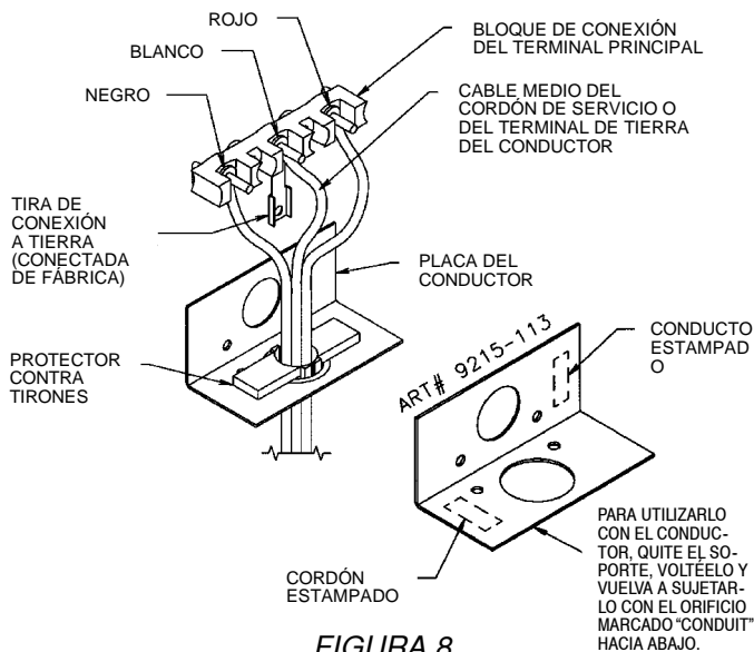
FIGURA 8 INSTALACIÓN ACEPTABLE DEL ENCHUFE DE 3 CABLES
