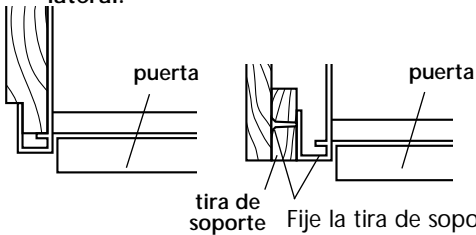
panel lateral empotrado fuera de la moldura lateral
