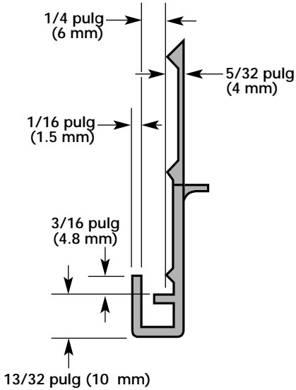
Vista de extremo de la moldura lateral
