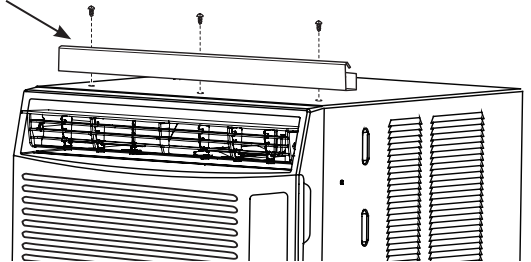
Riel de montaje superior
