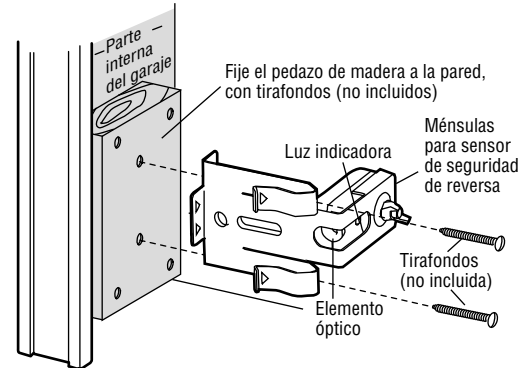
Figura 2 MONTAJE PARED (LADO DERECHO)
