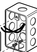
Figura 2 INSTALACIÓN PRECABLEADA
