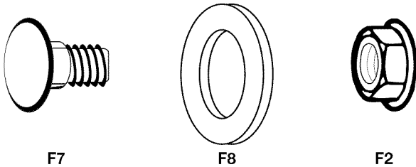
F7 Perno de carruaje (9) F2 Tuerca de reborde de 5/16" (9) F8 Arandela (9)
