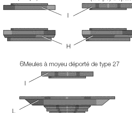
FIG. 15 Meules de type 1/41 d'une épaisseur de 3,17 mm (1/8 po) ou moins Meules de plus de 3,17 mm (1/8 po) d'épaisseur
