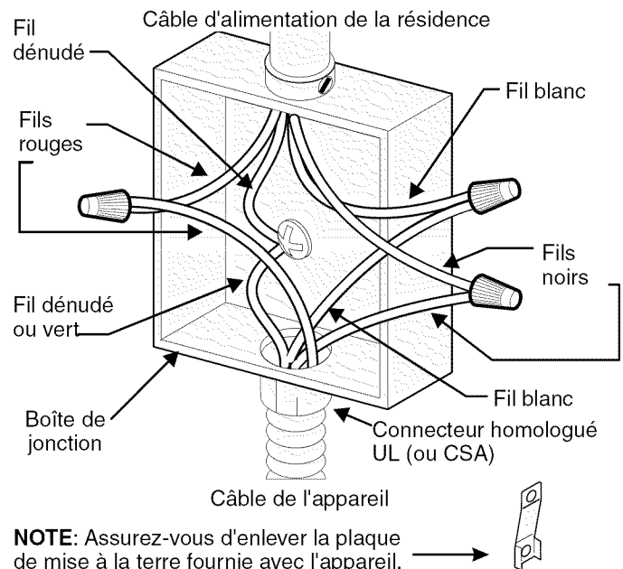
Figure 11 BOÎTE DE JONCTION À 4 FILS - MISE À LA TERRE
