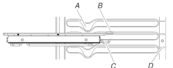
A. Encoche en "V" B. Glissières de grille C. Crochet de l'échelle D. Échelle
