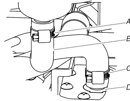
A. Abrazadera ajustable para manguera, de 7/8" B. Tubo de desagüe (del depósito de hielo a la bomba de desagüe) C. Abrazadera ajustable para manguera, de 7/8" D. Entrada del depósito de la bomba de desagüe
