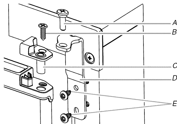
A. Axe de la charnière
