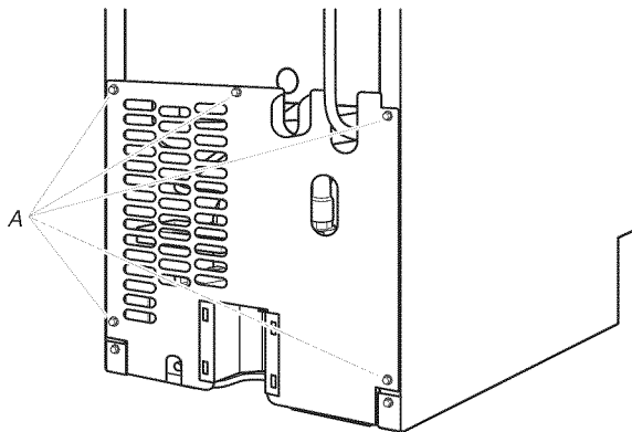
A. Emplacement des vis
