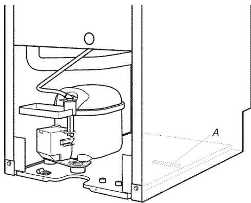
A. Encoche de la patte de montage
