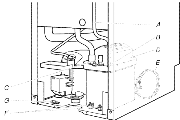
A. Tubo de ventilación B. Abrazadera para manguera, de 5/8" C. Tubo de descarga de la bomba de desagüe D. Bomba de desagüe E. Cable eléctrico de la unidad de la fábrica de hielo F. Tornillos de montaje de la bomba N° 8-32 x 3/8" G. Cable eléctrico de la bomba de desagüe, abrazadera y tornillo
