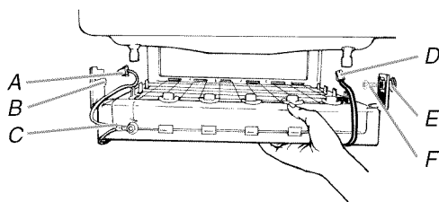
A. Arnés de la rejilla de corte
