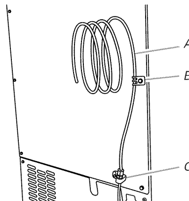
C. Bride pour tuyau d'admission d'eau et connecteur à la canalisation d'alimentation en eau
