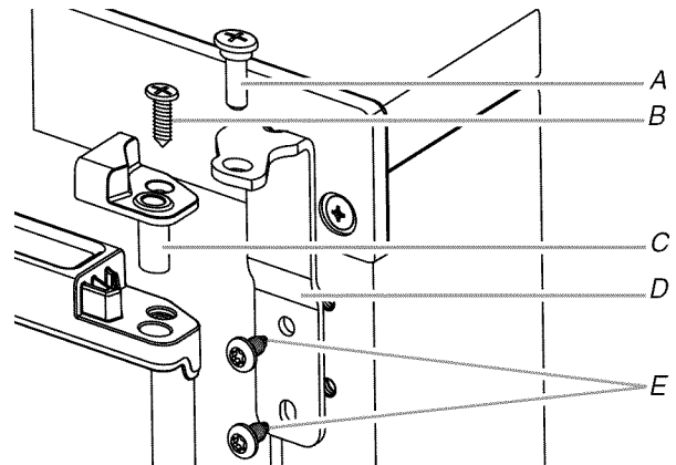
A. Pasador de la bisagra
