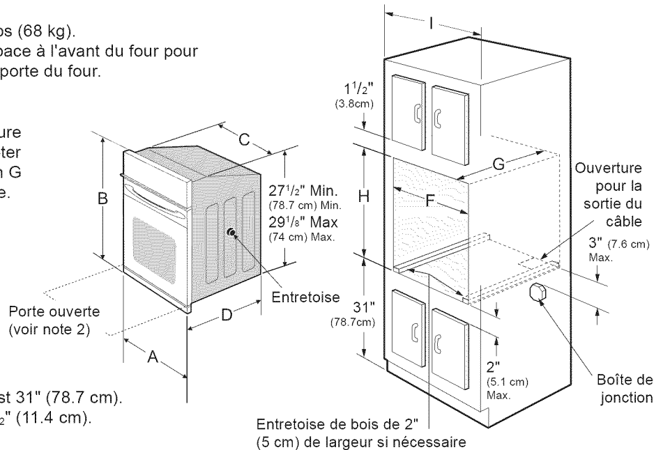
Figure 1 FOURS ENCASTRÉS SIMPLES 24" (Pour les fours encastrés doubles voir la figure 2)
