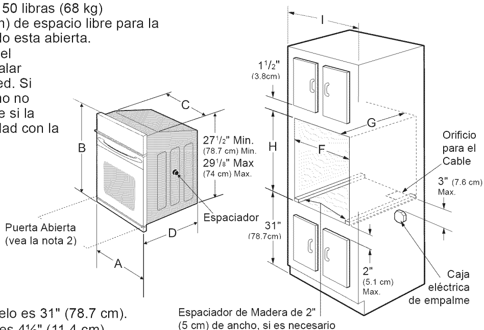
Figura 1 HORNO SENCILLOS DE PARED DE 24" (Para hornos dobles, ver la Figura 2)
